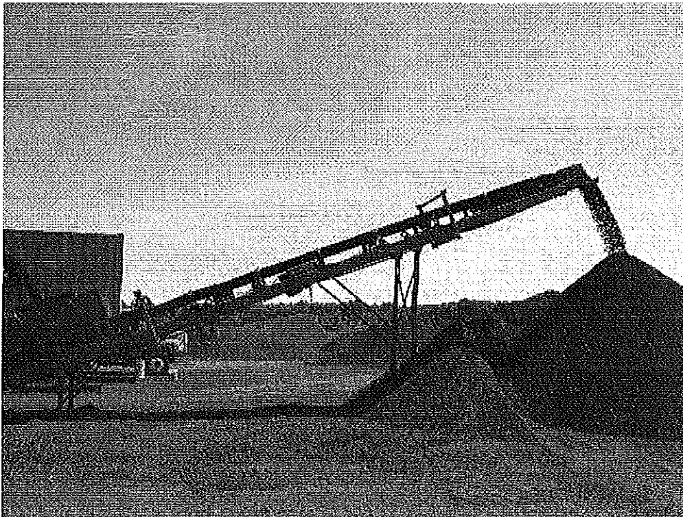
Image 4(2014_4) : Conveyor #1--1101
